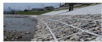
平铺式生态框护坡
